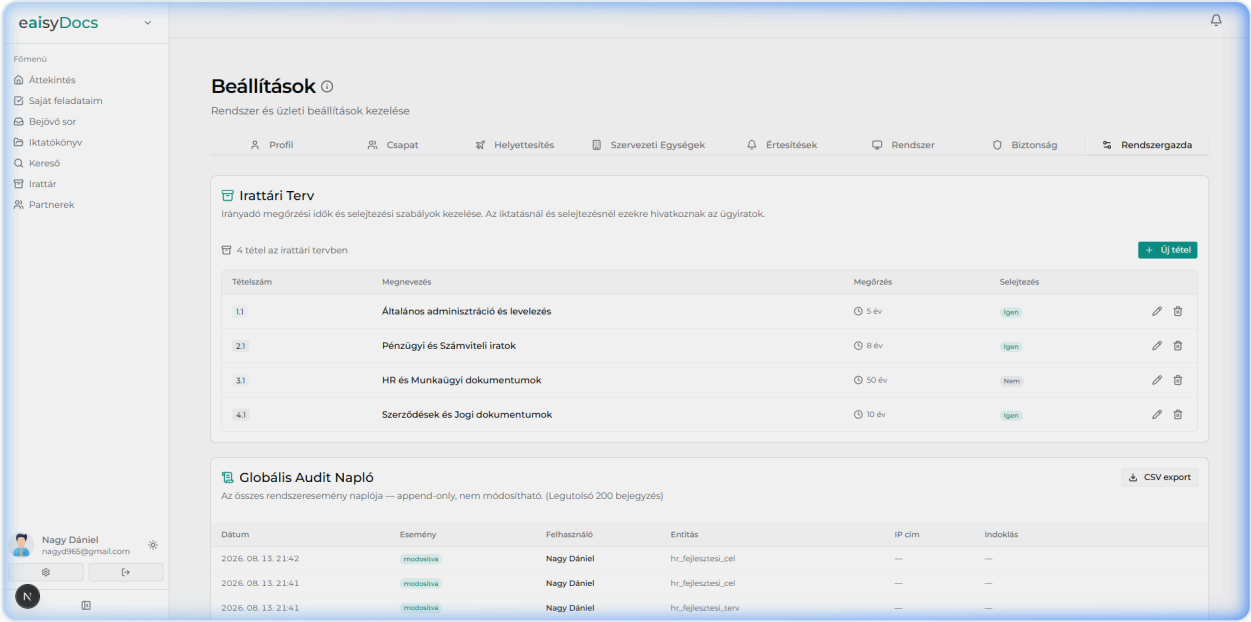
20. ábra: Rendszergazdai konfigurációs panel a szervezeti struktúra és irattári terv karbantartásához
